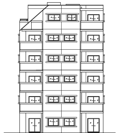
南立面図 S=1/300
