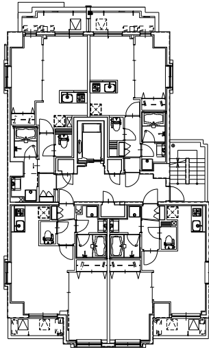
2~5階平面図 S=1/300
