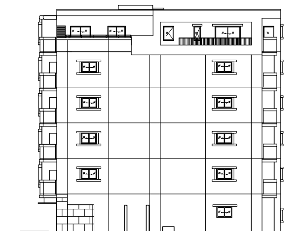
西立面図 S=1/300
