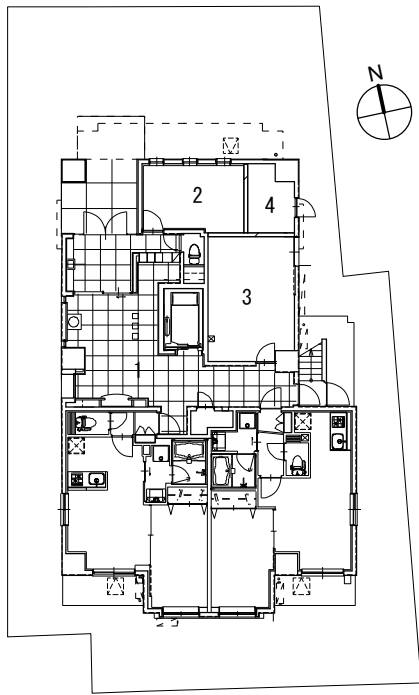
1階平面・配置図 S=1/300
