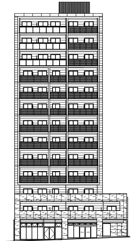
南立面図 S=1:400
