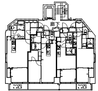
11~13階平面図 S=1:400
