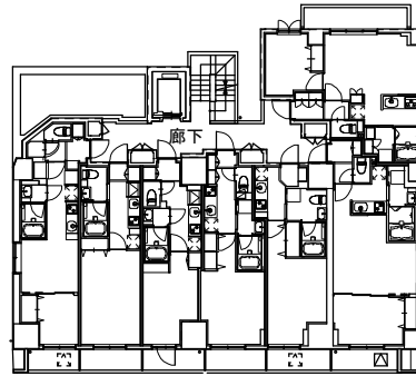
2階平面図 S=1:400
