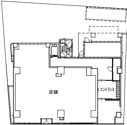
1階平面図 S=1:400
