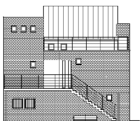
北立面図
