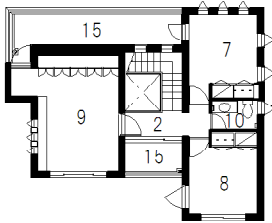
3階平面図
