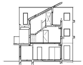
断面図 1/300
