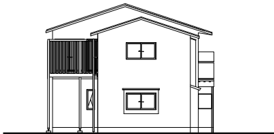
東立面図
