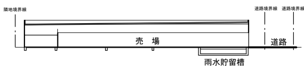
断面図-1
