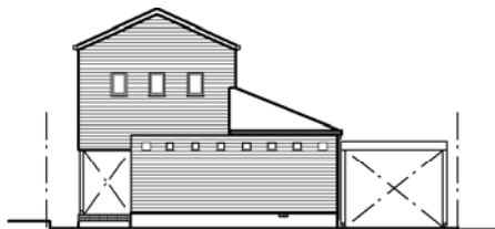
北立面図
