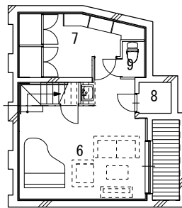
地下1階平面図
